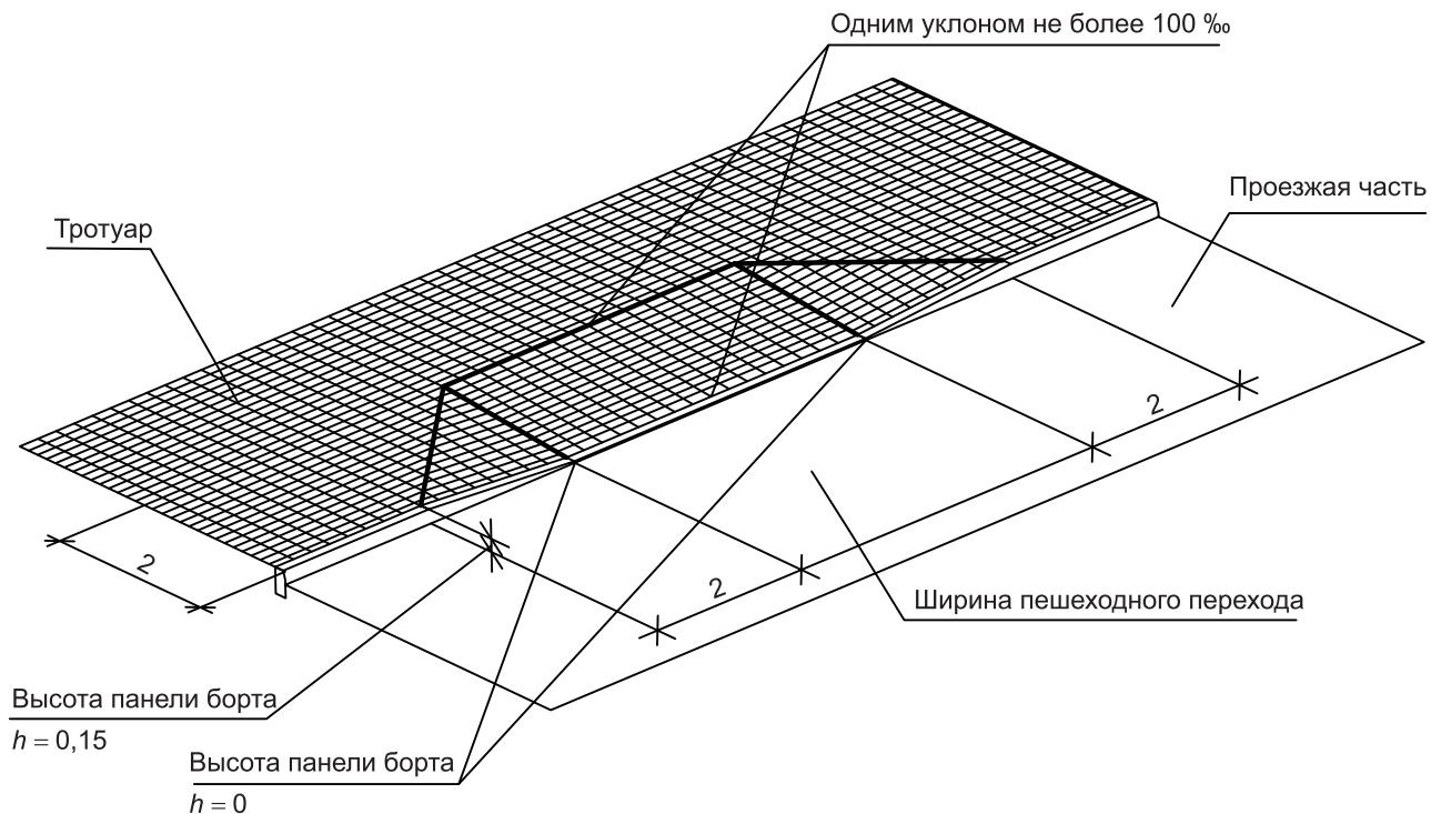
Рисунок Г.1 — Фрагмент устройства пониженного борта проезжей части на пешеходном переходе при отсутствии зеленой зоны и ширине тротуара 4,5 м и более
