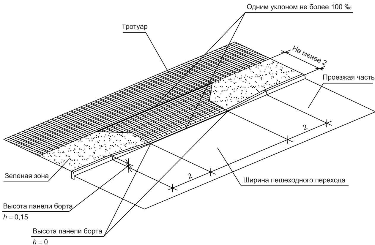
Рисунок Г.3 — Фрагмент устройства пониженного борта проезжей части на пешеходном переходе при наличии зеленой зоны
