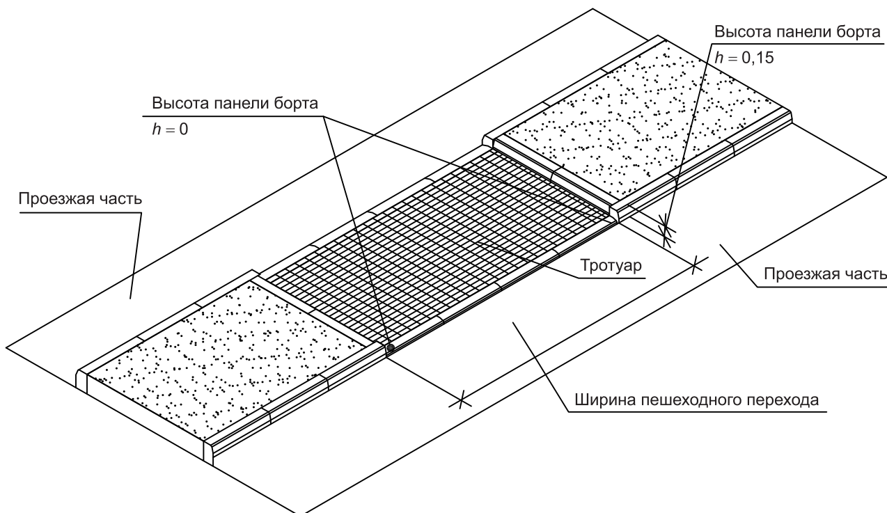
Рисунок Г.4 — Фрагмент устройства пониженного борта проезжей части на пешеходном переходе на разделительной полосе (островке безопасности), вариант 1
