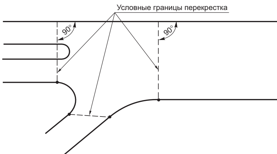
Рисунок В.2 — Определение условных границ перекрестков на примыканиях
