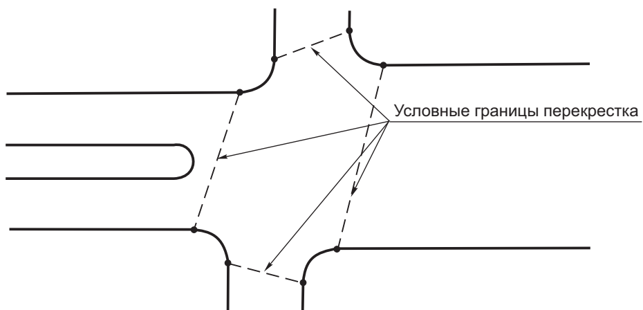
Рисунок В.1 — Определение условных границ перекрестков на пересечениях
