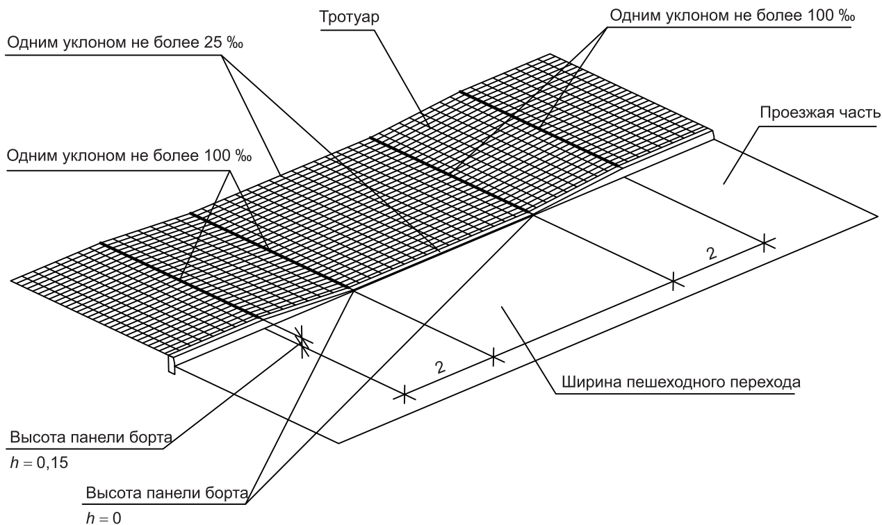
Рисунок Г.2 — Фрагмент устройства пониженного борта проезжей части на пешеходном переходе при отсутствии зеленой зоны и ширине тротуара менее 4,5 м
