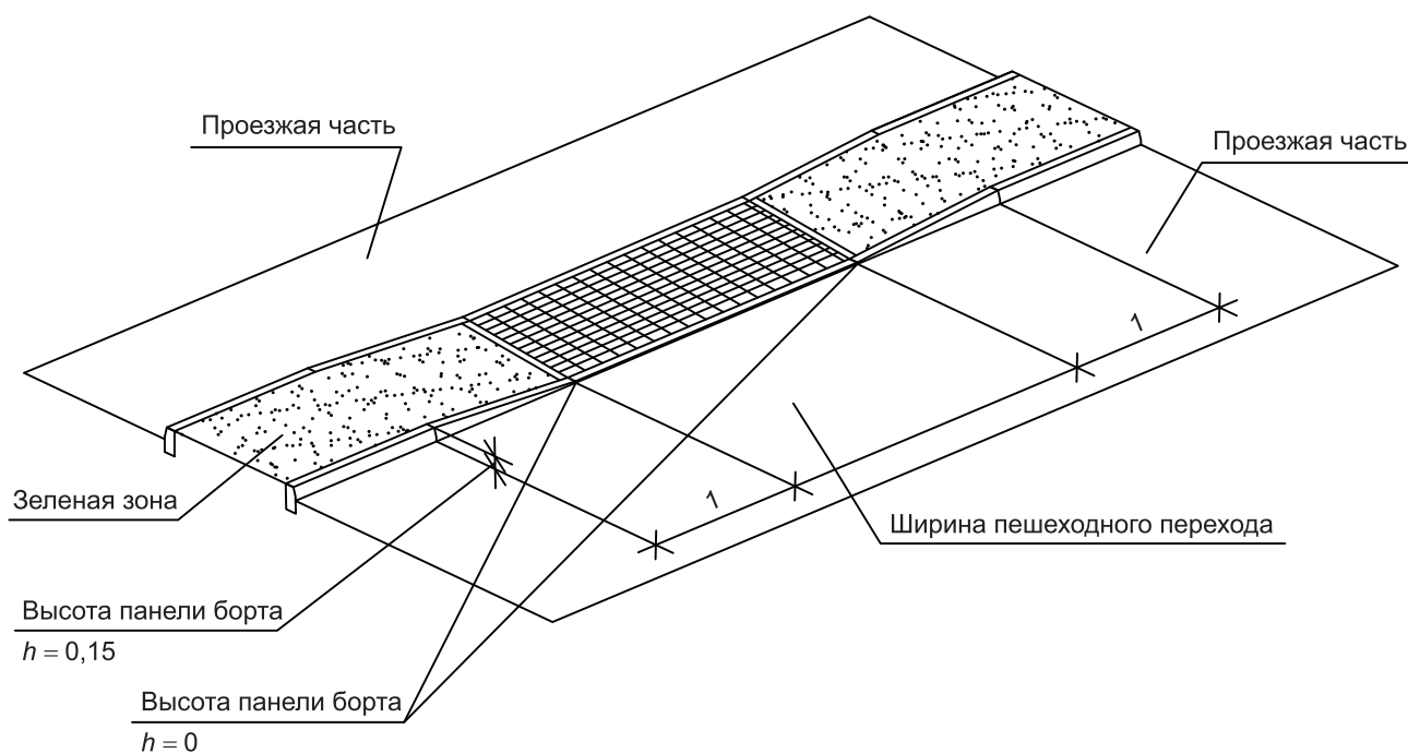
Рисунок Г.5 — Фрагмент устройства пониженного борта проезжей части на пешеходном переходе на разделительной полосе (островке безопасности), вариант 2
